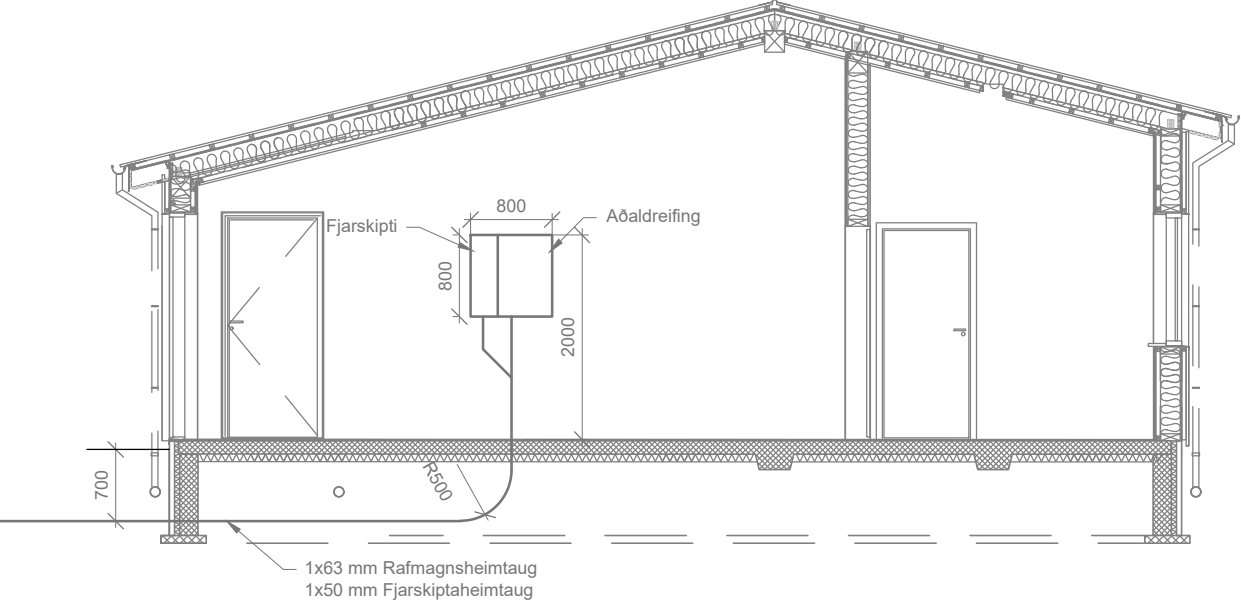
Snið 1:50
